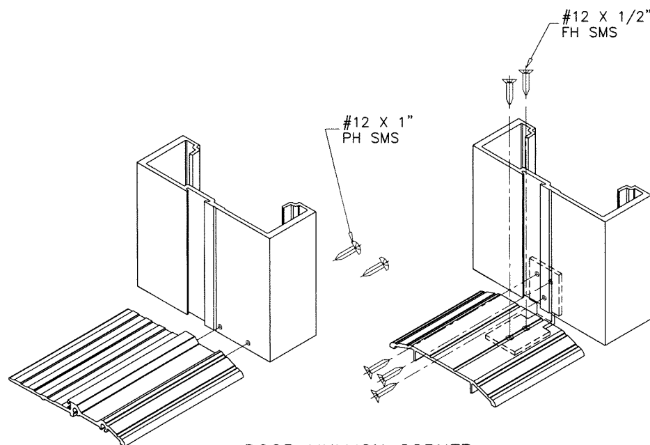
DOOR MULLION CORNER
